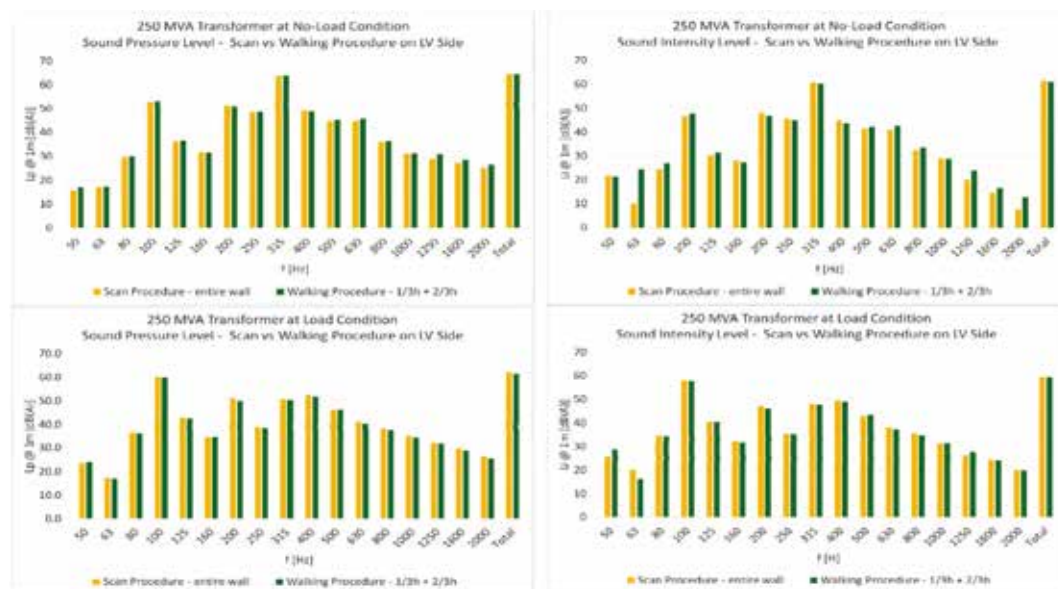
Rys. 3. Porównanie pomiarów hałasu przeprowadzone przy użyciu dwóch różnych procedur pomiaru ciągłego „walk-along” vs. „scanning”
